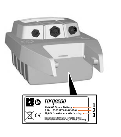
Fig. 37: Typeplaatje accu
