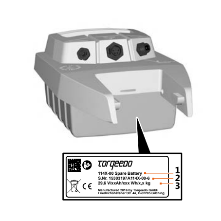
Fig. 2: Typeskilt batteri
