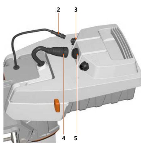
Fig. 28: Elektriske forbindelser
