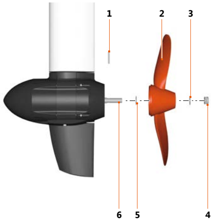
Fig. 33: Propelfastgørelse Travel 503/1003
